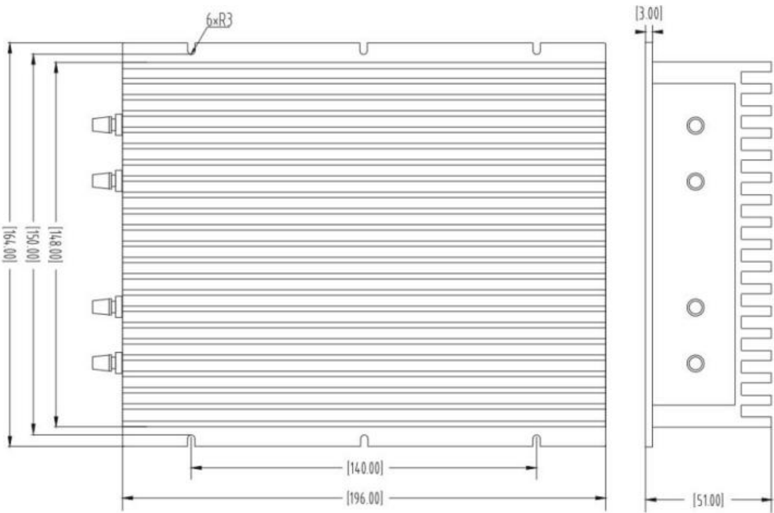
机械尺寸图（单位：mm）
